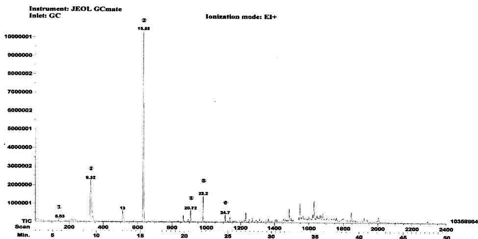
Fig.2. 精油カクラリセージ Salvia sclarea のGC-MSクロマトグラム [myrcene(1)、linalool(2)、linalool acetate(3)、geranyl acetate(4)、 \beta -caryophyllene(5)、amorpha-4,7-diene(6).]
