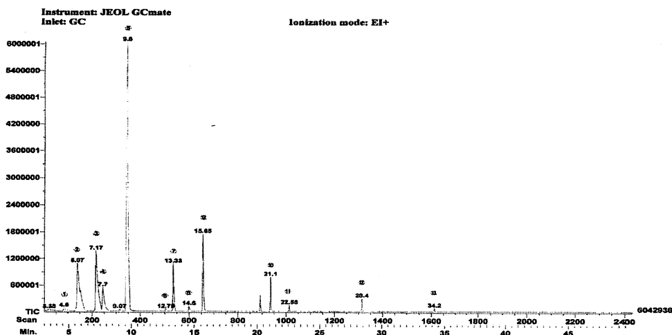
Fig.6. 精油ネロリ Citrus aurantium のGC-MSクロマトグラム [α-pinene(1)、β-pinene(2)、limonene(3)、(E)-β-ocimene(4)、linalool(5)、terpinen-4-ol(6)、dihydro carveol (7)、citronellol(8)、geraniol(9)、2-epi-α-funebrene(10)、β-caryophyllene(11)、(E)-nerolidol(12)、and nerolidyl acetate(13).]
